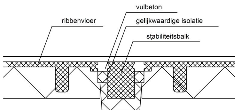
betonbalk tussen ribbenelementen
