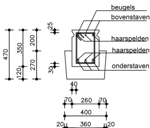
doorsnede
