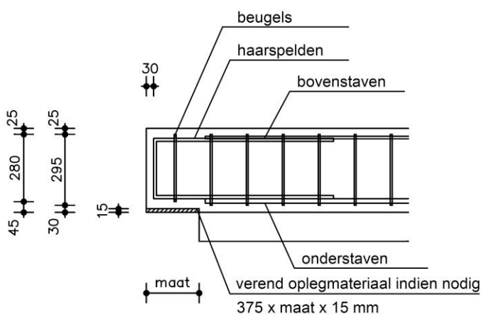
langsdoorsnede
