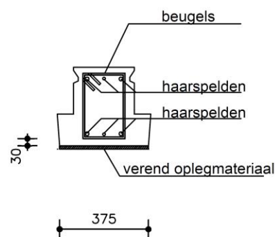
doorsnede t.p.v. oplegging
