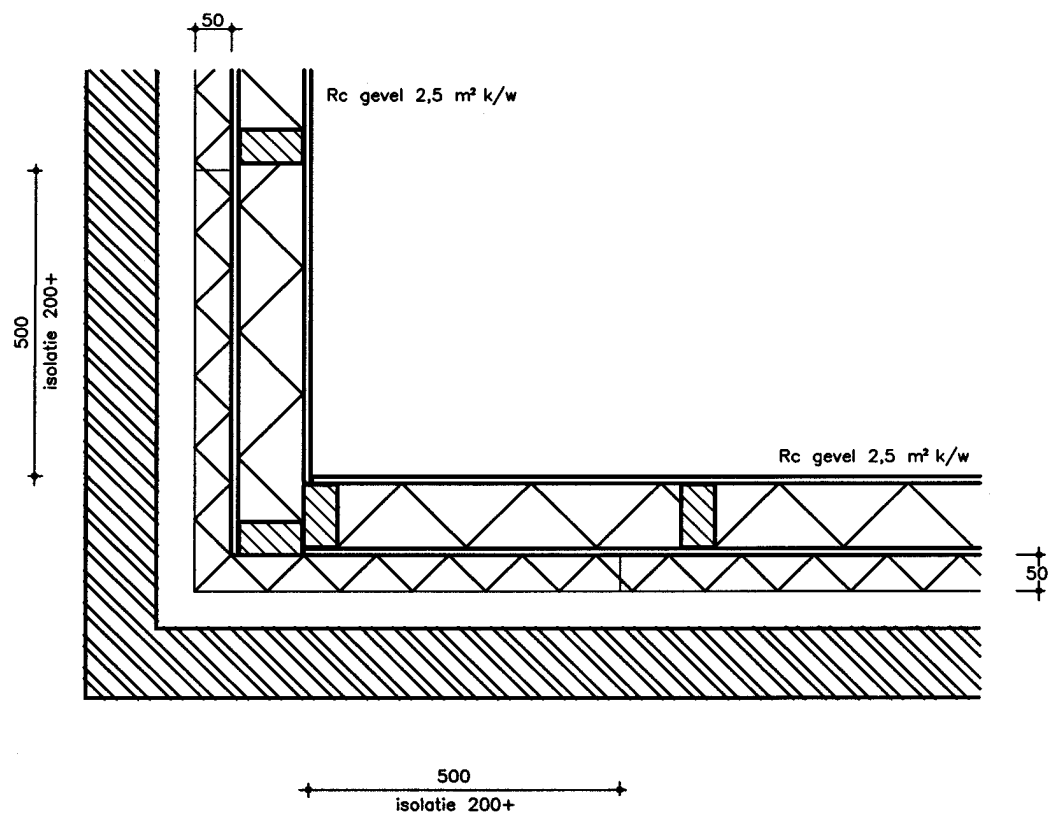
Doorsnede 2/BG
